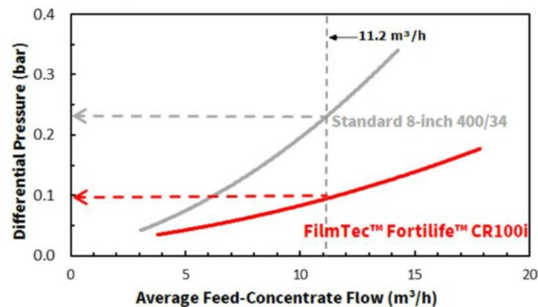
Abbildung 1: Elementdifferenzdruck als Funktion der Durchflussrate für FilmTec™ Fortilife™ CR100i-Elemente im Vergleich zu Standard-BWRO-Elementen
